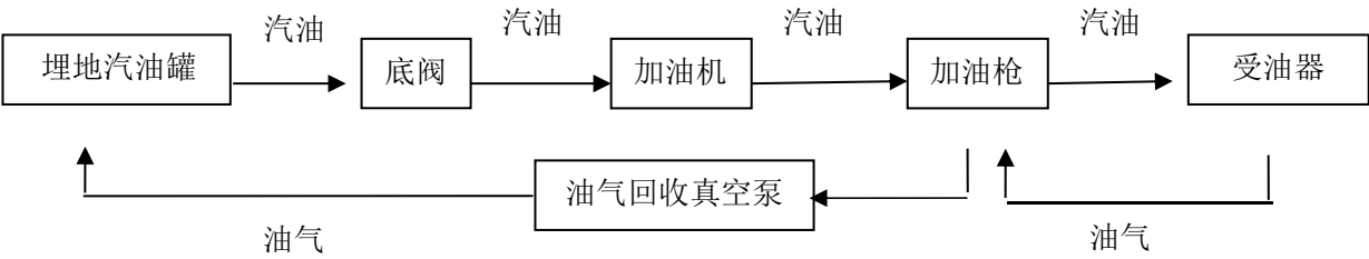
图 2.7-3 乙醇汽油加油工艺流程简图
